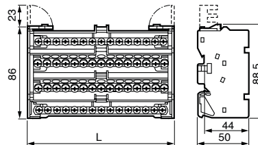
Tetrapolares 100 - 125 A
