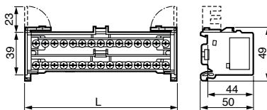
Bipolares 100 - 125 A
